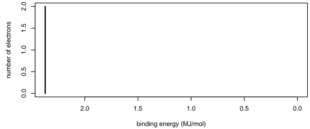
helium
