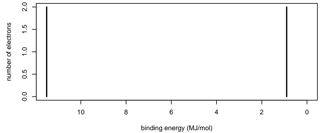
beryllium
