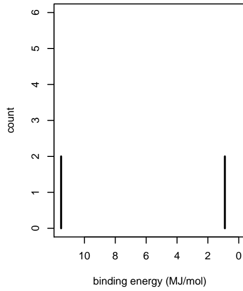
beryllium
